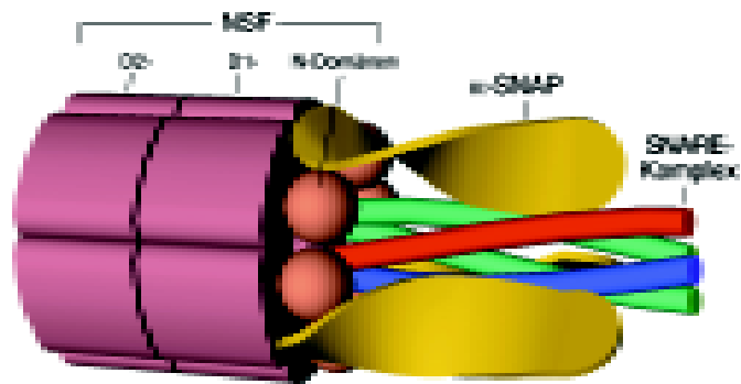
Abb. 5: Modell des SNARE-Komplexes mit gebundenem \alpha -SNAP und NSF vor dem Disassembly. Die N-terminale Spitze des Komplexes ist möglicherweise im „Loch“ der D1-D2-Domäne von NSF arretiert. Die N-Domänen könnten dann bei ATP-Hydrolyse eine (relativ zur D1-D2-Domäne) Rotationsbewegung ausführen, die durch \alpha -SNAP hebelartig auf die Mitte des Komplexes übertragen wird.
