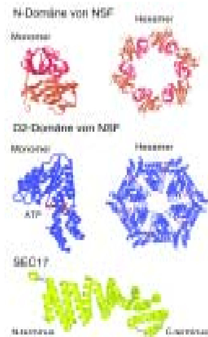
Abb. 4: Kristallstrukturen des SNAP-Proteins aus Hefe (Sec17p) [18] sowie der D2 [14-15] und N-Domäne von NSF [16-17]. Die D2-Domäne wurde als Hexamer kristallisiert, sie enthält ein ATP-Molekül (rot), das aber nicht hydrolysiert wird. Das \gamma -Phosphat des ATP-Moleküls bindet jeweils an eine Seitenkette der benachbarten Untereinheit. Dies erklärt, warum ATP für den Zusammenhalt des Hexamers benötigt wird.
