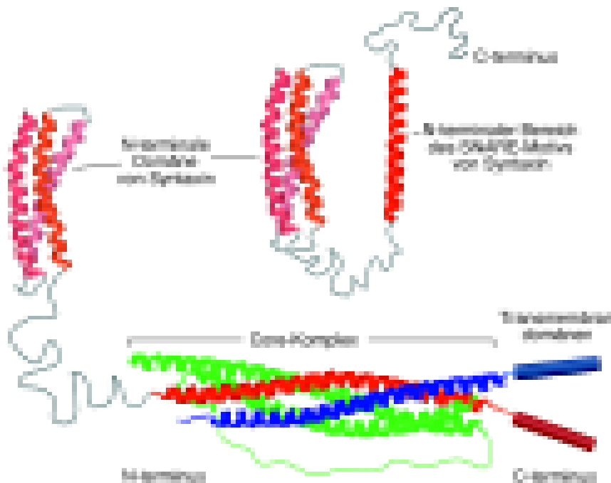
Abb. 2: Vergleich der offenen und geschlossenen Konformation von Syntaxin. Gezeigt ist die Kristallstruktur des neuronalen Core-Komplexes [1] sowie die NMR-Struktur der N-terminalen Domäne von Syntaxin1 [4]. Im SNARE-Komplex ist die N-terminale Domäne frei beweglich und durch eine flexible Verbindung unbekannter Struktur mit dem Core-Komplex verbunden. In der geschlossenen Konformation bindet die N-terminale Domäne an den N-terminalen Bereich des SNARE-Motivs, welches auch hier eine \alpha -helikale Struktur hat. Der C-terminale Teil des Motivs ist dagegen nicht strukturiert. Die Transmembrandomänen sind als Zylinder dargestellt, Bereiche unbekannter Struktur als Linien.
