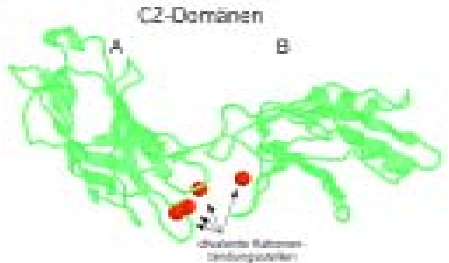
Abb. 3: Kristallstruktur der C2-Domänen von Synaptotagmin [23]. Die roten Kugeln deuten die Position der divalenten Kationen an. Ca^{2+} -Bindung ist nicht mit einer meßbaren Konformationsänderung verbunden. Die Bindung dieser Domänen an Phospholipide bzw. SNAREs wird vermutlich ausschließlich durch die Fixierung der positiv geladenen Ionen an der Protein-Oberfläche bewirkt („electrostatic switch“).
